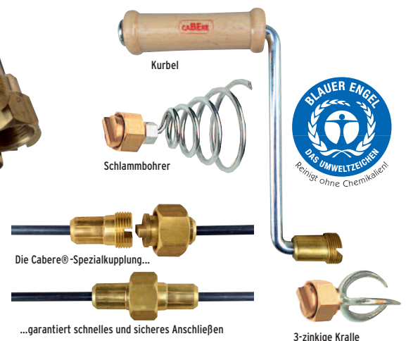
3-zinkige Kralle
